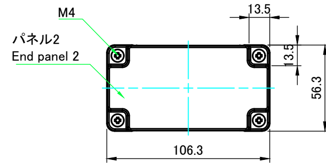
A-A ( 1 : 2.5 )
