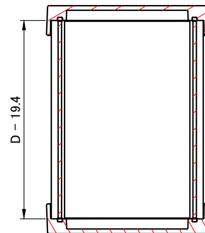
C-C ( 1 : 2.5 )
